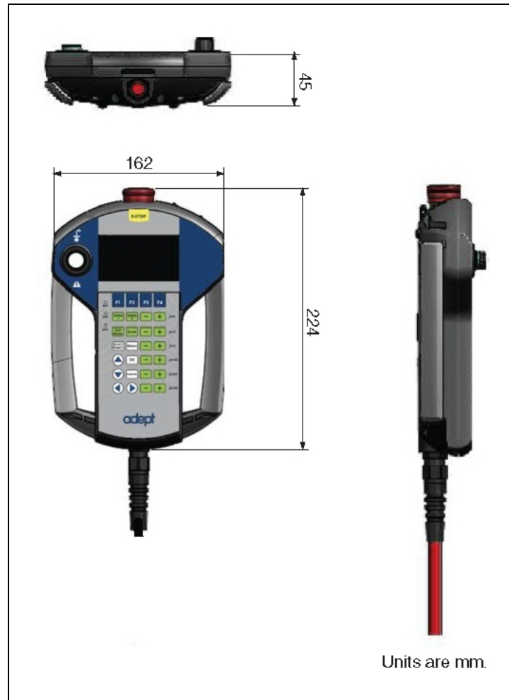
Figure 6-1. T20 Pendant Dimensions
