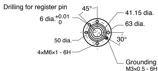
Flange
